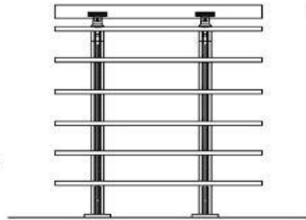
PESPA 001 TUBULAR KIT Ø40 CORNER 45°
